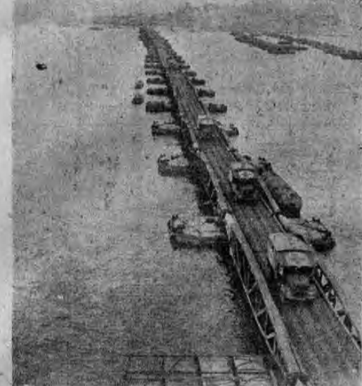
Este puente, extraordinariamente flexible, está compuesto de docenas de pequeños puentes de acero colocados sobre flotadores lo cual le permite subir o bajar según la marea. Este producto del ingenio de las fábricas británicas, forma parte de esa gran invención conocida como "puertos prefabricados" que se han empleado en la invasión de Europa.
